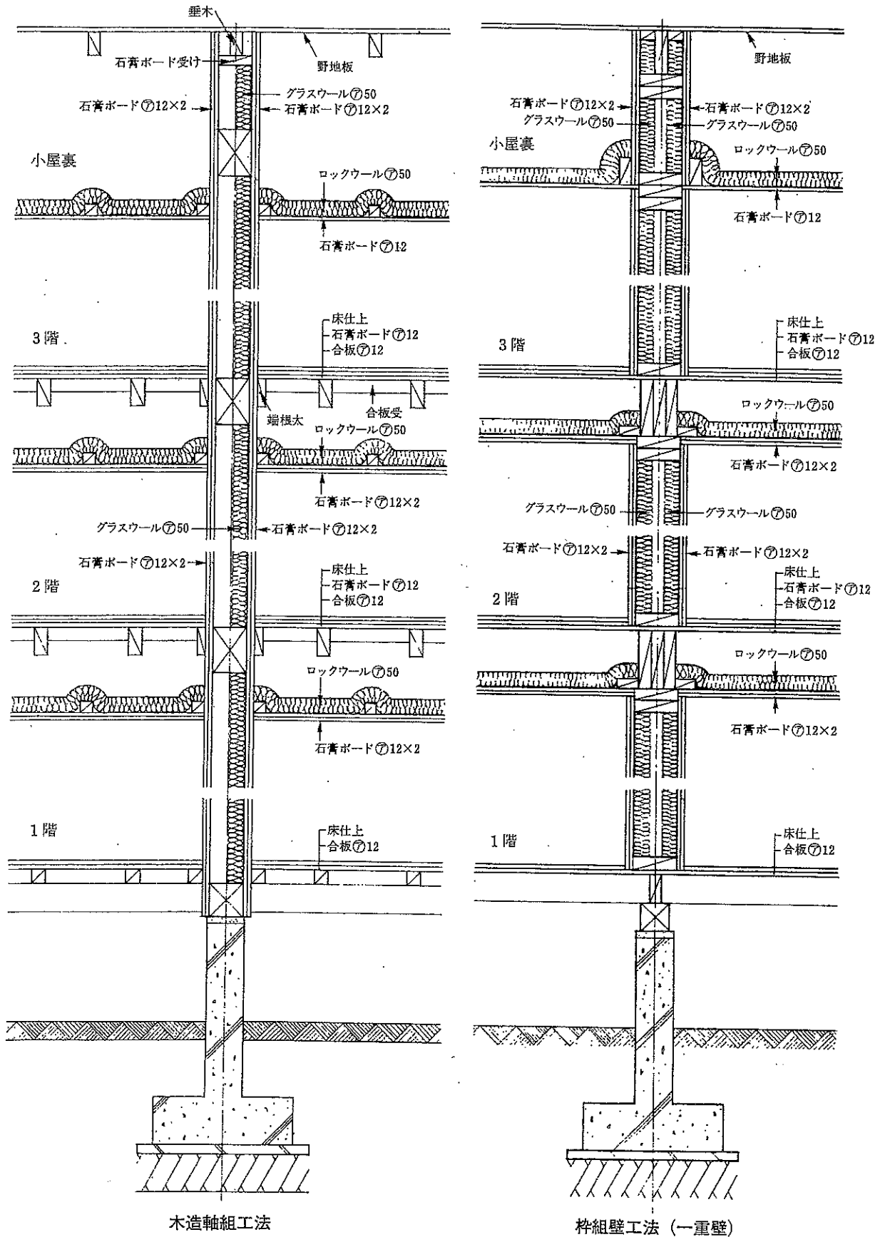
図2.5-41 界壁の例(1)
